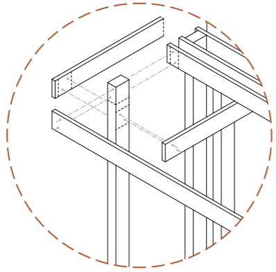
Holzbalkenverbindung mit Schrauben
