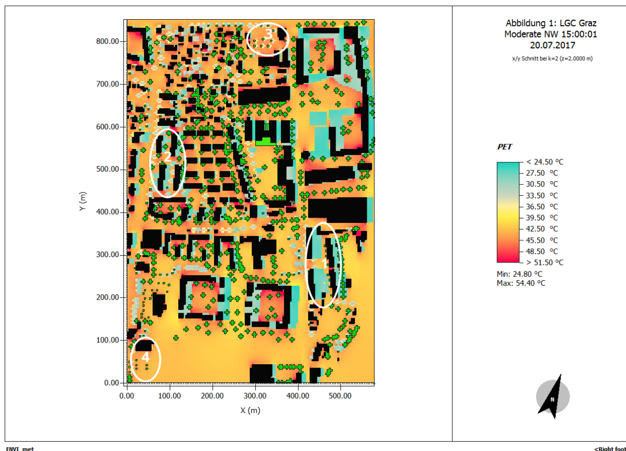
Abbildung 16 - Simulationsergebnisse für die Flächenanteile mit thermophysiological Belastung des LGC Projektgebietes in der MODERATE Variante
