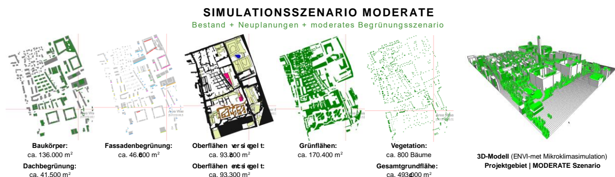
Abbildung 15 Simulationsszenario MODERATE LGC Graz | Dekomposition Typologien | generiertes 3D Modell
